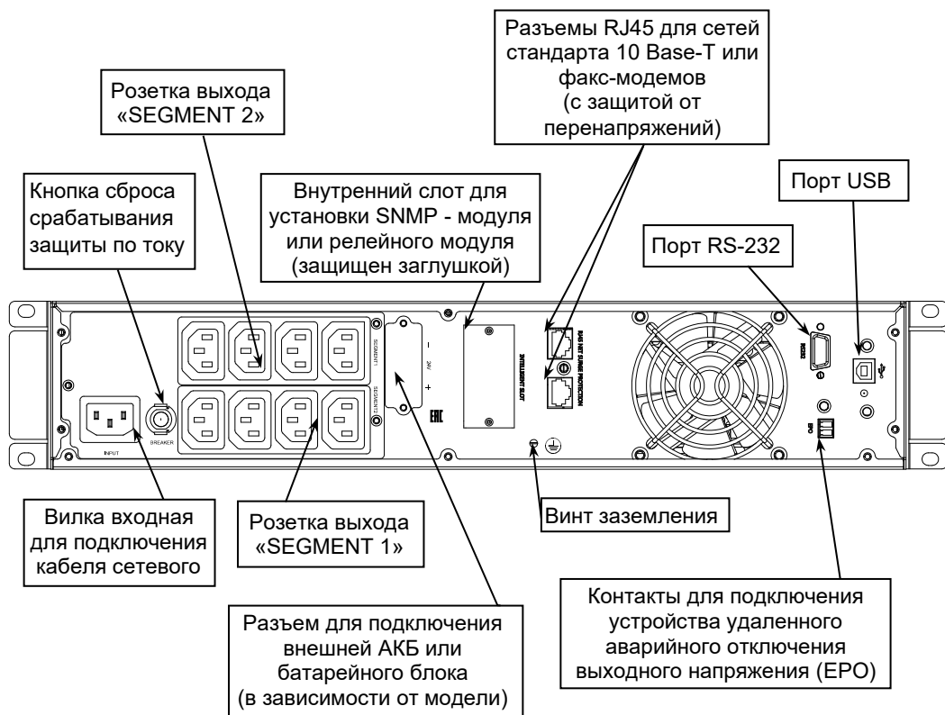
Рисунок 3 – Общий вид задней панели SKAT-UPS 1000-RACK-ON-2x9-E P3, SKAT-UPS 1000-RACK-ON-E P3, SKAT-UPS 1500-RACK-ON-3x9-E P3, SKAT-UPS 1500-RACK-ON-E P3
