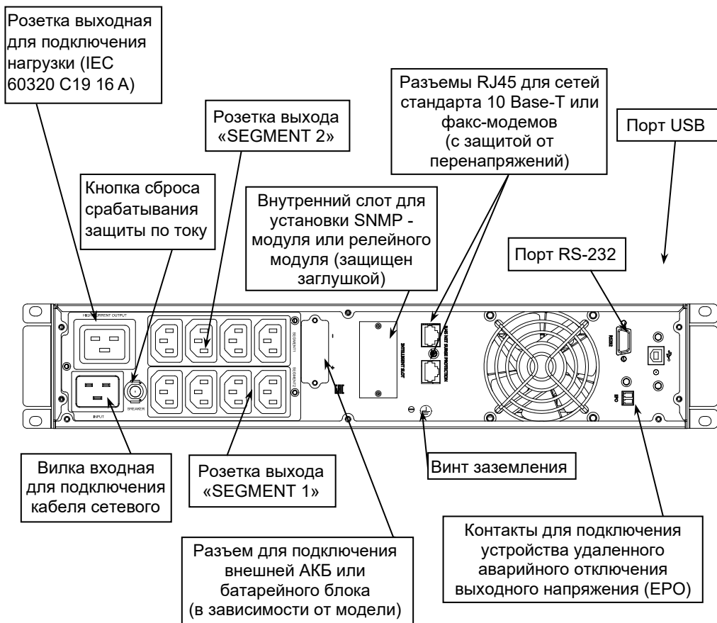
Рисунок 7 – Общий вид задней панели SKAT-UPS 3000-RACK-ON-6x9-E P3, SKAT-UPS 3000-RACK-ON-E P3
