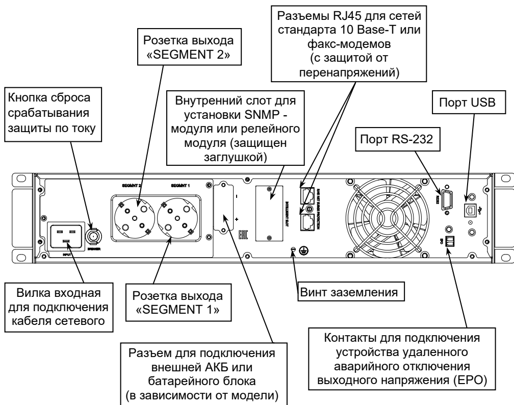
Рисунок 4 – Общий вид задней панели SKAT-UPS 2000-RACK-ON-4x9 P3, SKAT-UPS 2000-RACK-ON P3
